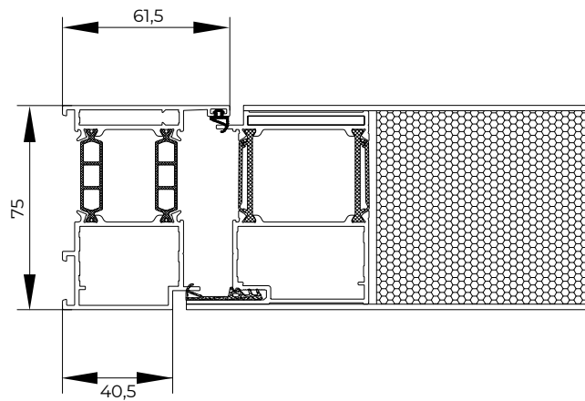
Ajtó keresztmetszete
