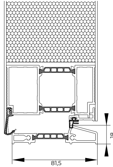
Küszöb
