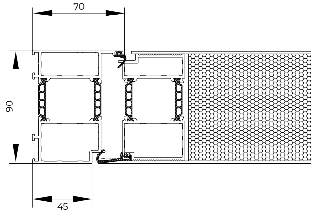
Ajtó keresztmetszete
