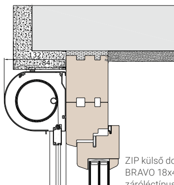
ZIP külső doboz BRAVO 18x44 záróléctípussal
