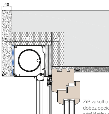
ZIP vakolható külső doboz tolókeretes rovarhálójával és 18x44 záróléctípussal
