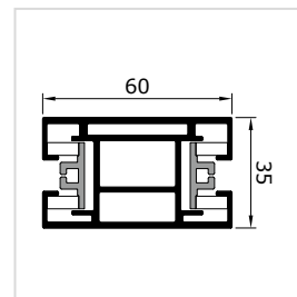
FS ZT60V Önhordó ikersín
