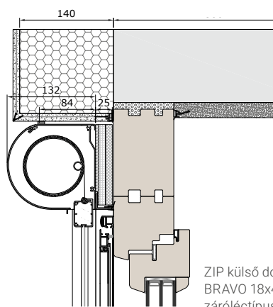
ZIP külső doboz BRAVO 18x44 záróléctípussal
