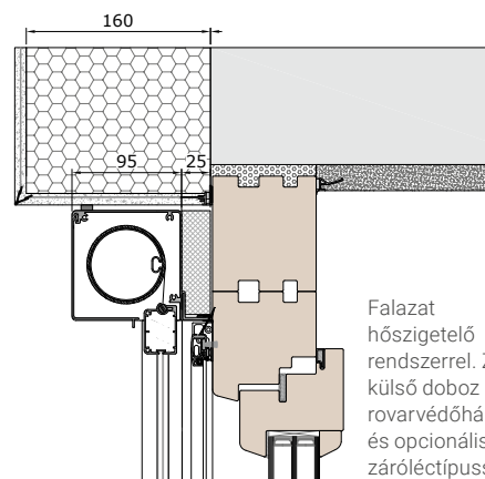
ZIP külső doboz 18x44 záróléctípussal
