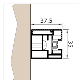
FS ZG37VS vezetősín, kávára rögzíthető szerkezet
