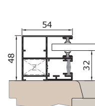
KR54V vezetősín
