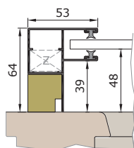
Termikusan leválasztott K53VT vezetősín
