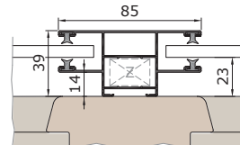
KE85V vezetősín
