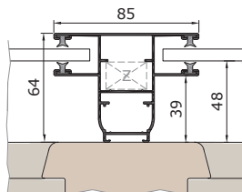
KD85V vezetősín
