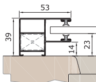
KE53V vezetősín felújításhoz
