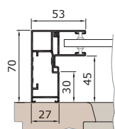
Vezetősín KD53SA
