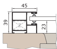
KF45V vezetősín
