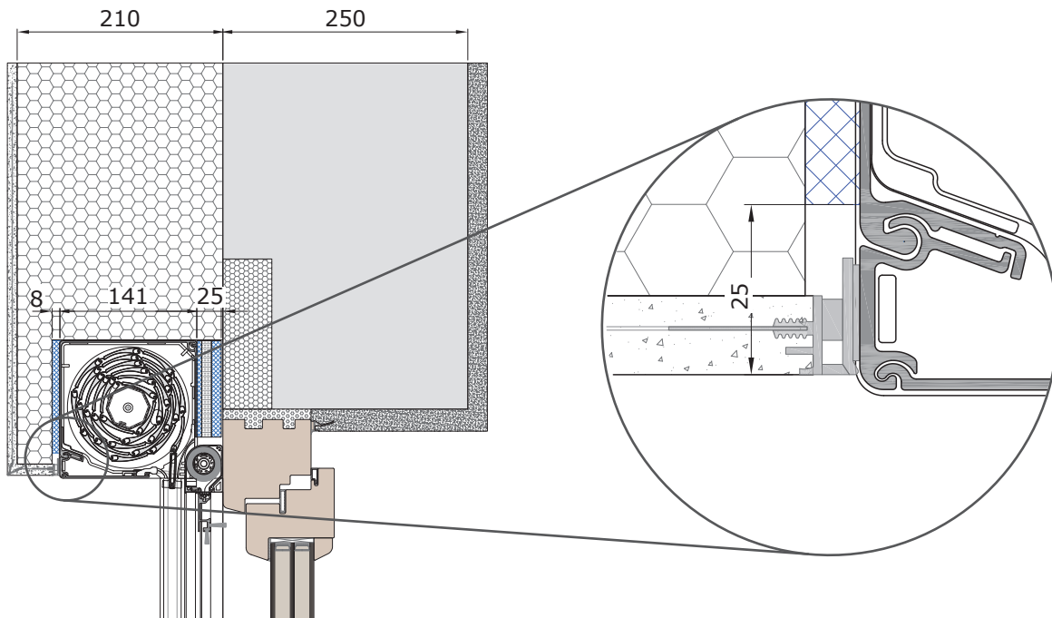
Hőszigetelésbe építve és üregszigeteléssel. VORO WDVS rolós szűnyoghálóval.
