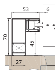
ED53V vezetősín
