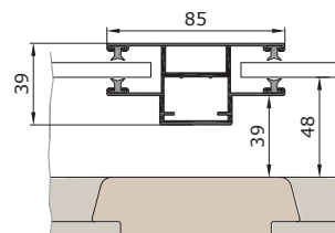
Ablakkeret öntartó vezetősínnel
