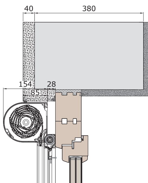
Tokmagasítással. VORO BRAVO rolós szűnyoghálóval.
