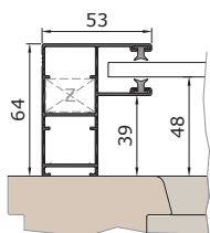
KD53V vezetősín
