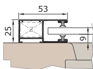
K53V vezetősín
