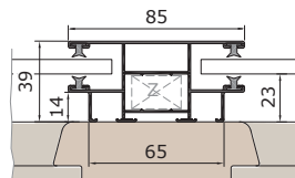
KF85V vezetősín
