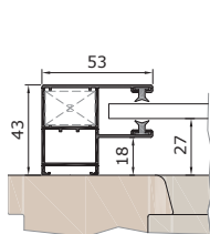
KA53V vezetősín
