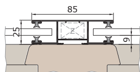
K85V vezetősín
